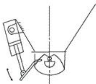
B 操纵料斗闸式闸门开关
